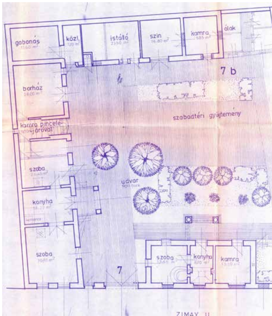
A Zimay László utca 7. szám alatti porta felmérési rajza – a tervezett néprajzi gyűjtemény helyszíne (Kecskeméti népi műemléki vizsgálata, Kecskeméti Katona József Múzeum)
