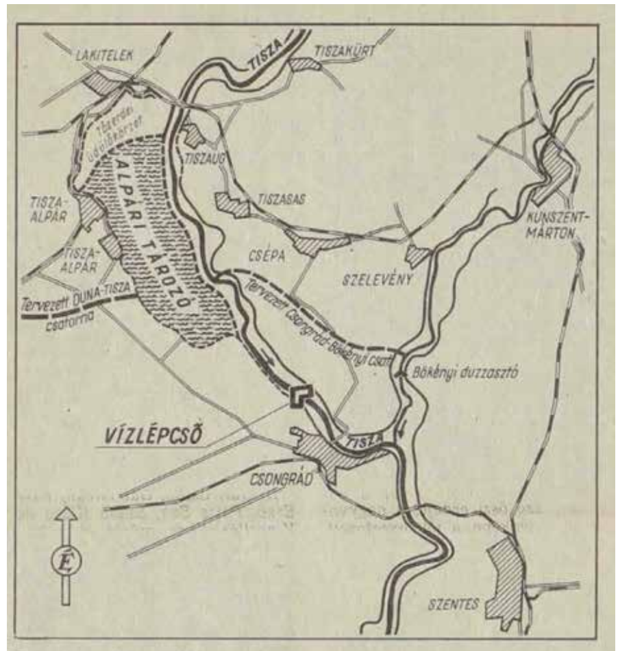
A csongrádi vízlépcső tervrajza
