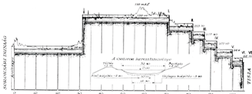
A kivitelezésre elfogadott magasvezetésű csatorna tervrajza
