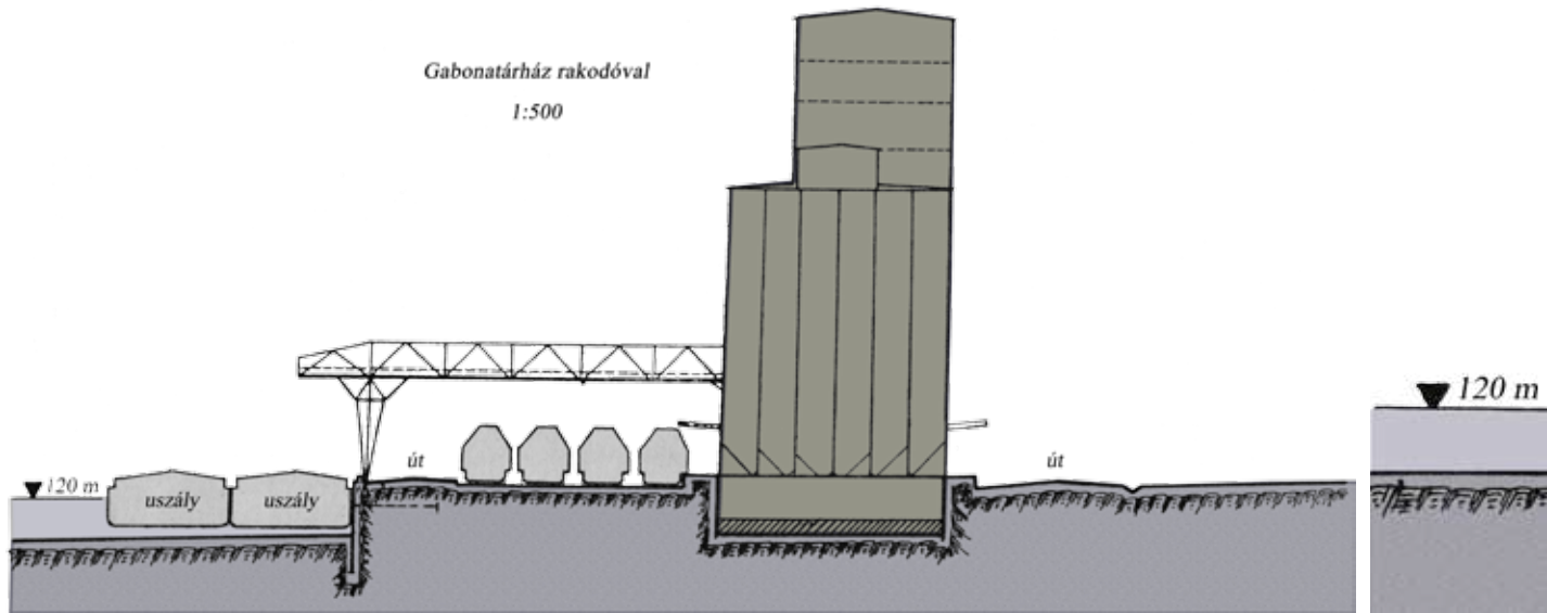
A tervezett gabonatóró tervrajza
