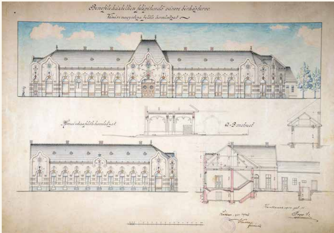
Papp Sándor: „Bene-féle háztelken felépítendő városi bérház terve” (1904. július 10., Magyar Nemzeti Levéltár Bács-Kiskun Megyei Levéltára)
