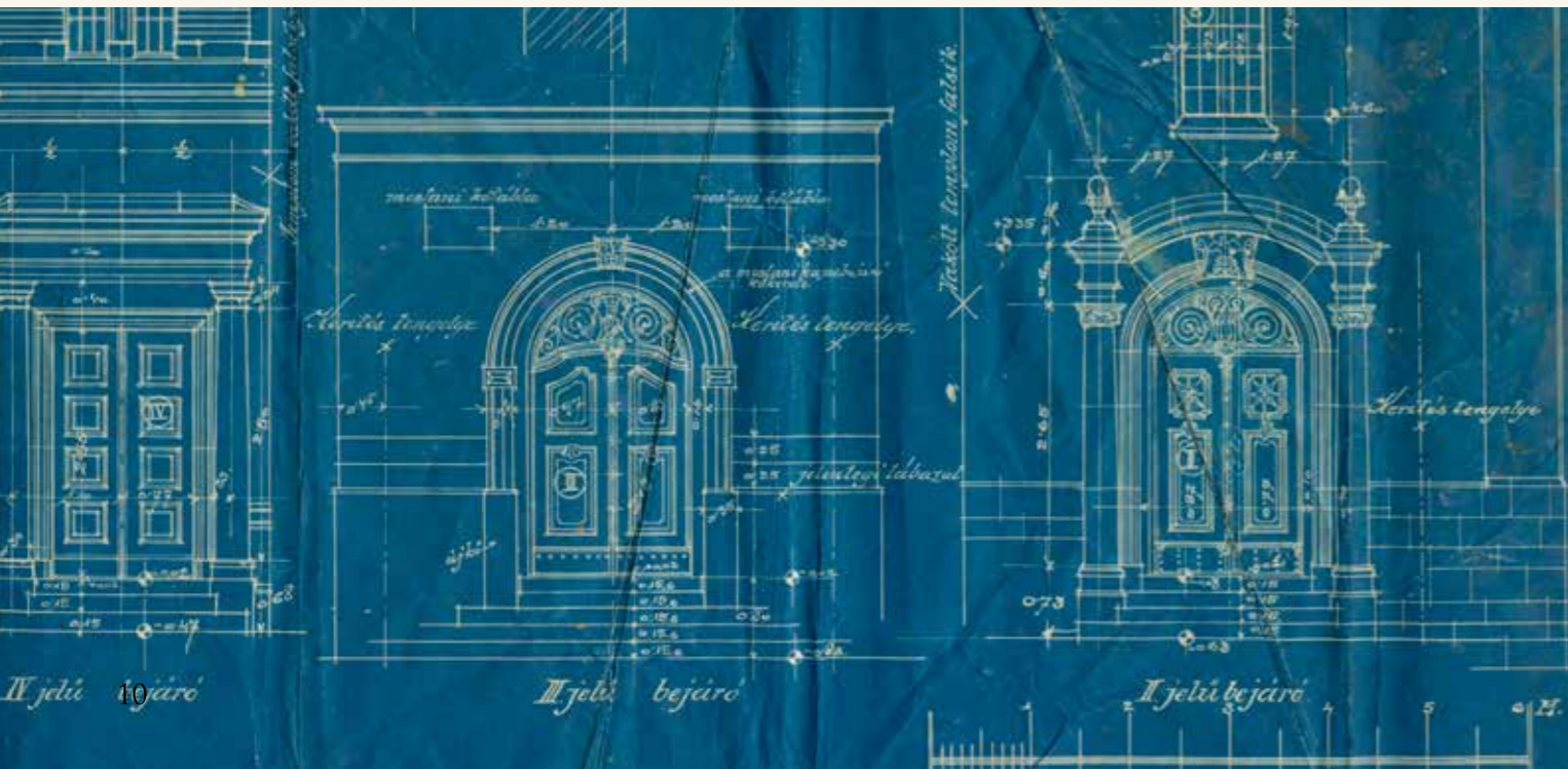
A református templom 1913-as, Takáts László által tervezett átalakításának homlokzati tervrajza. A közepén látható kapuzat az előcsarnoké, rajta feltüntetve a kerítés kapujából odakerülő részletekkel (Kecskeméti Református Egyházközség Könyvtára és Levéltára)
