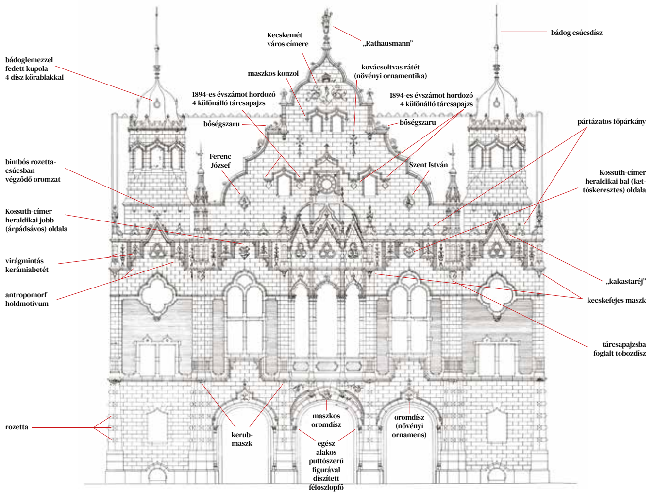
Bádó-, kerámia- és műkö díszek a Városháza főhomlokzatának középrizalitján (egy 1893-as tervrajz felhasználásával készítette: ifj. Gyergyádesz László és Olajosné Nagy Nikolett Vivien)
