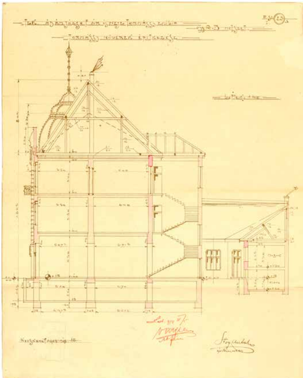
Stoy Antal: A-B metszet, „Tek. Ádám József úr és neje Tormássy Emília, Tormássy nővérek építkezése”, 1914. márc. 15. (Forrás: MNL BKML)
