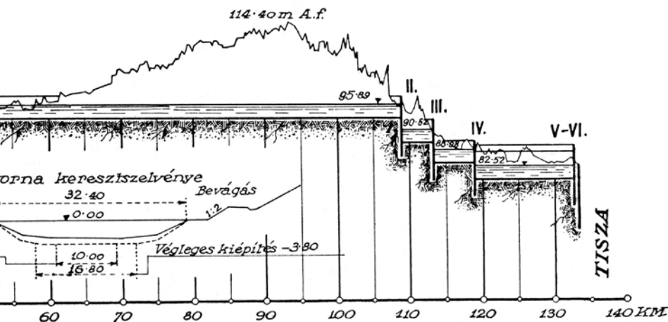
Egy Dunaharaszti és Csongrád közötti mélybevágású csatorna tervrajza
