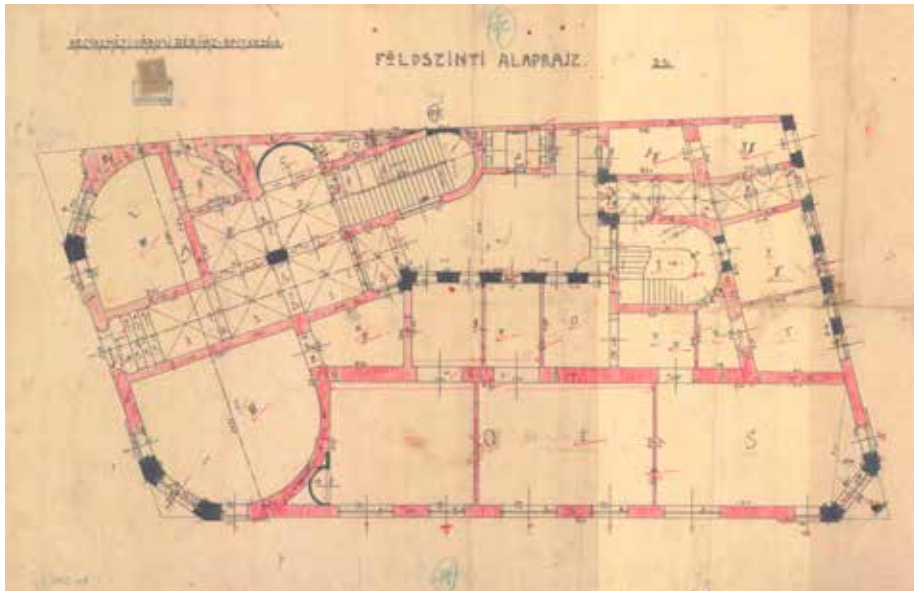
„Kecskemét Város Központi Iktató Hivatalába” 1903 októberében, az épület használatbavételi engedélyezési eljárása után leadott földszinti alaprajz (Magyar Nemzeti Levéltár Bács-Kiskun Megyei Levéltára)
