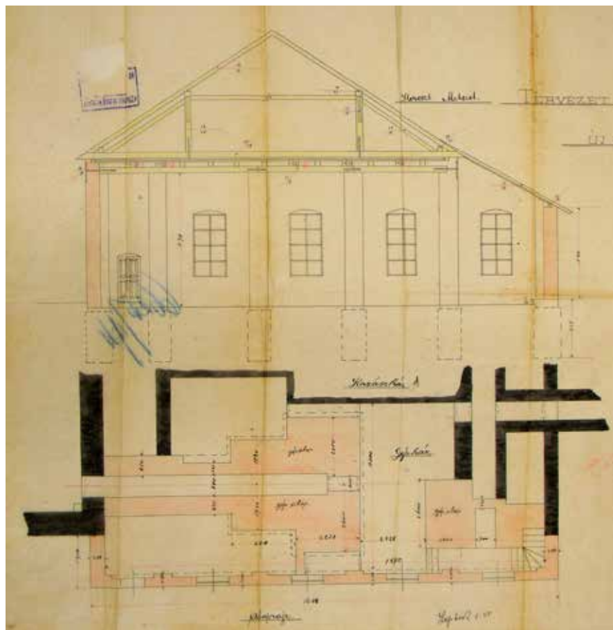
A gépház keresztmetszeti tervrajza (1894)
