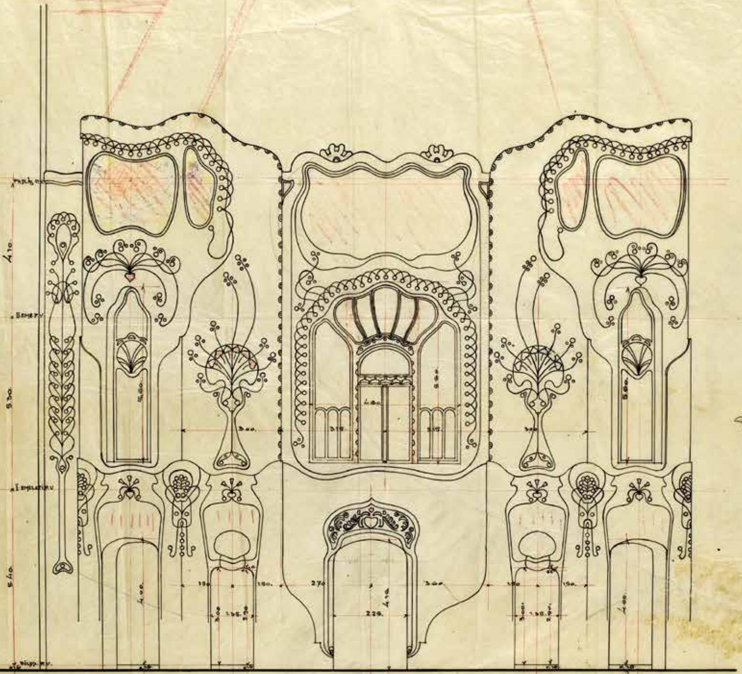
Márkus Géza tervrajza a Cifrapalota Klapka utcai homlokzatához, 1902. november 3. (Magyar Nemzeti Levéltár Bács-Kiskun Megyei Levéltára)
