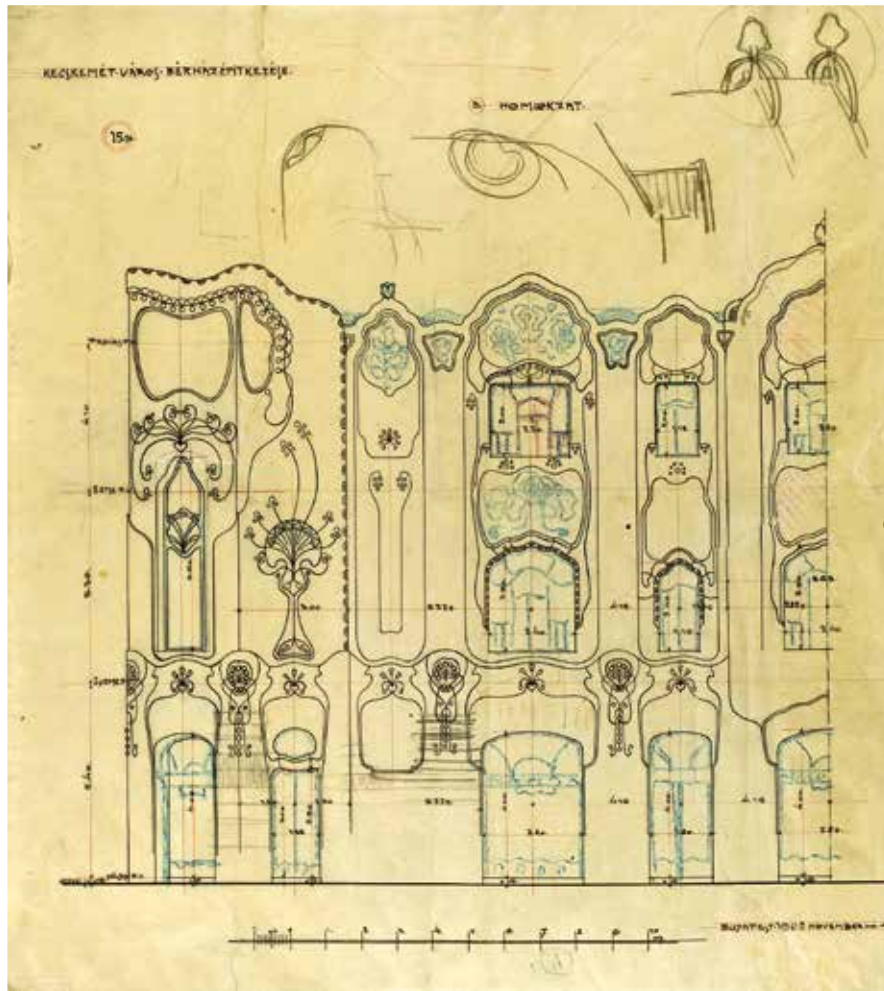
Márkus Géza tervrajza a Cifrapalota Rákóczi úti homlokzatához, 1902. november 4. (Magyar Nemzeti Levéltár Bács-Kiskun Megyei Levéltára)
