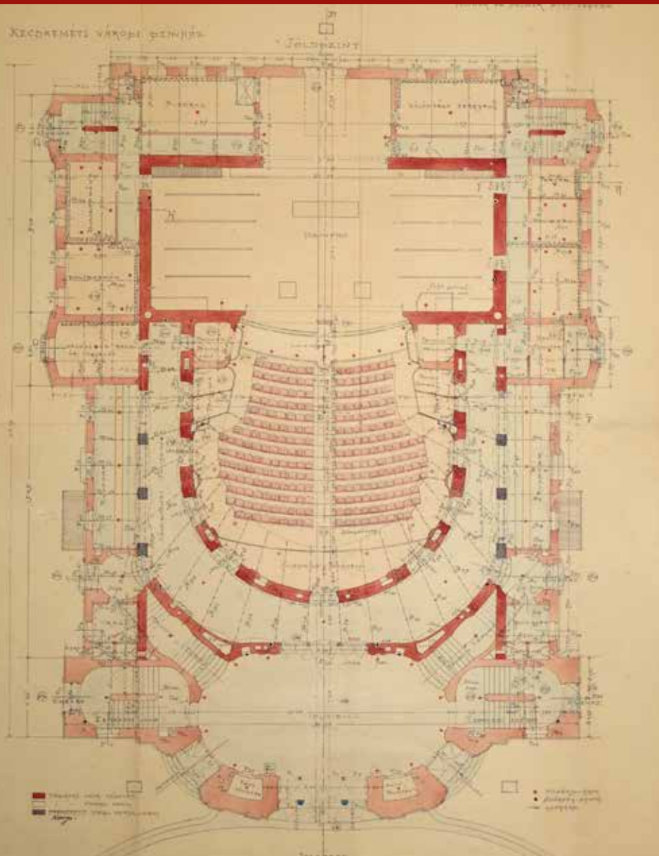
A földszint tervjaja (Fellner és Helmer, 1895, Magyar Nemzeti Levéltár Bács-Kiskun Megyei Levéltára)
