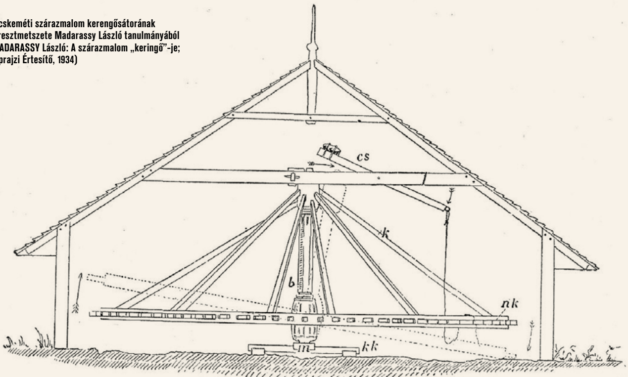
1. ábra. kk = koszorúkötés, m = medvegerenda, b = bálvány, j = járom, cs = csapógerenda, k = küllő, nk = nagykerék.
