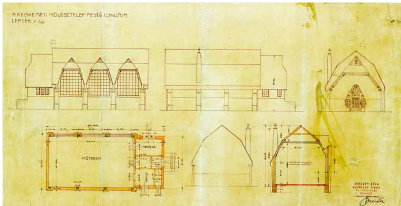
Janszky Béla és Szivessy Tibor: A festőiskola tervrajza, 1910 (Magyar Nemzeti Levéltár Bács-Kiskun Megyei Levéltára)
