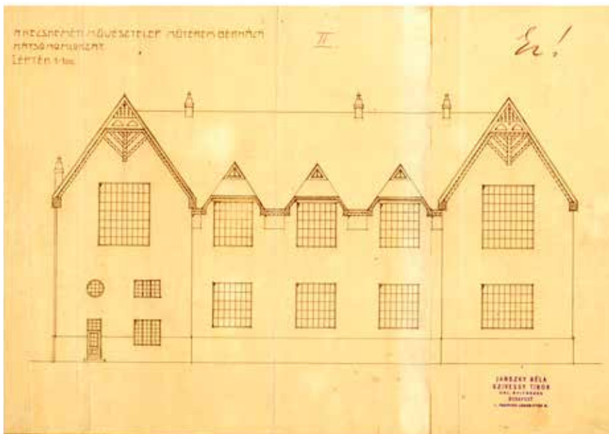
Jánszky Béla és Szivessy Tibor: A központi műterembérház hátsó homlokzatának tervrajza, 1910 (Magyar Nemzeti Levéltár Bács-Kiskun Megyei Levéltára)
