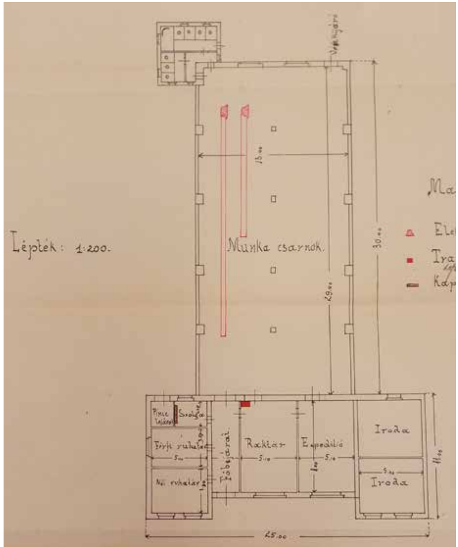
A Schiffer Cipőgyár tervrajza (MNL BKML)
